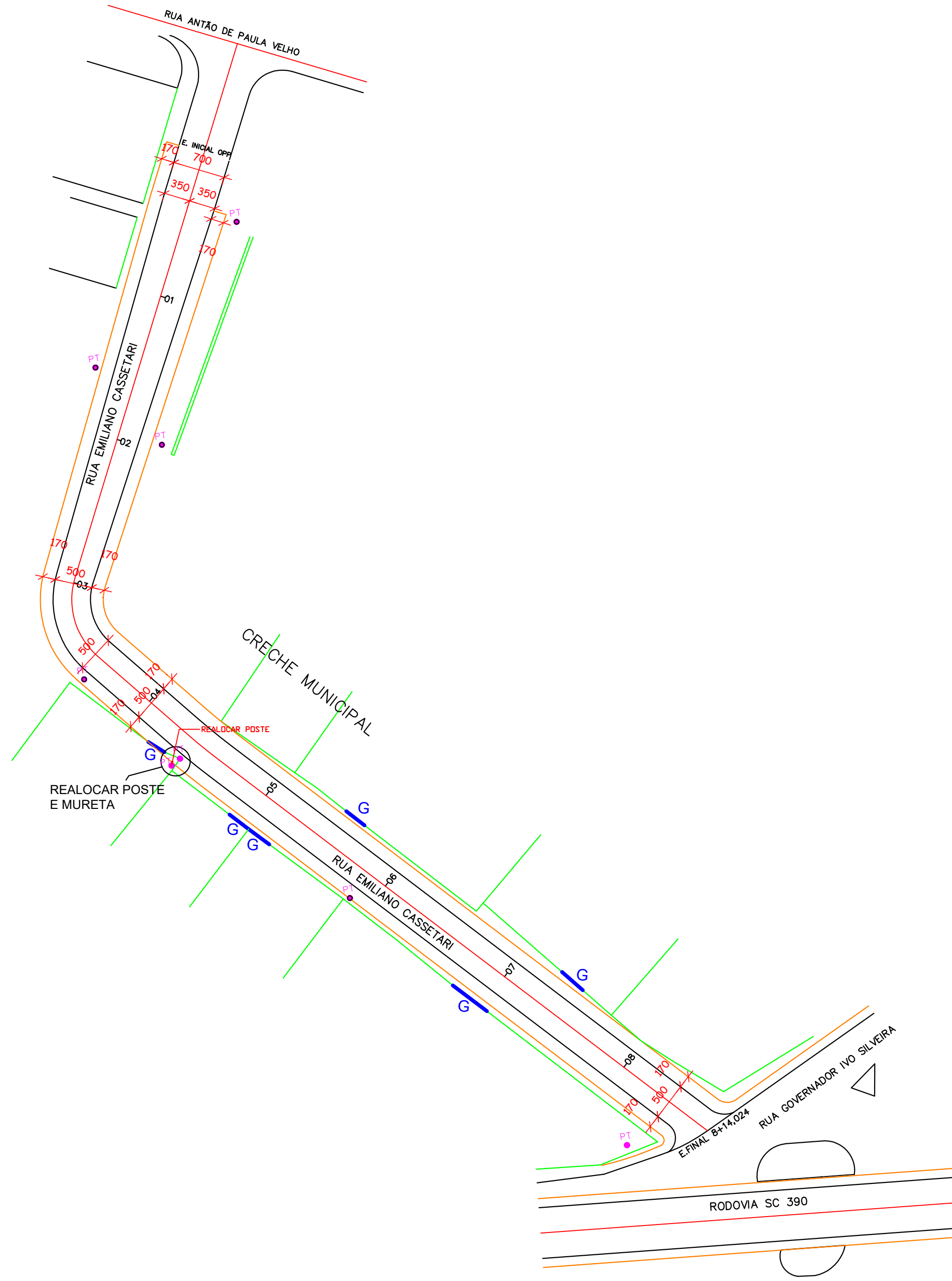
PROJETO GEOMÉTRICO E ESTAQUEAMENTO ESCALA 1:500
