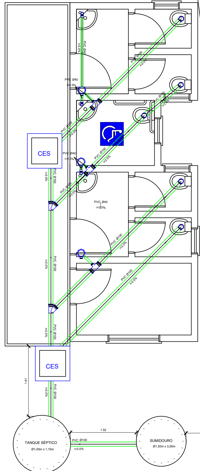
PLANTA BAIXA DE INSTALAÇÕES HIDROSANITÁRIAS ESCALA - 1/50
