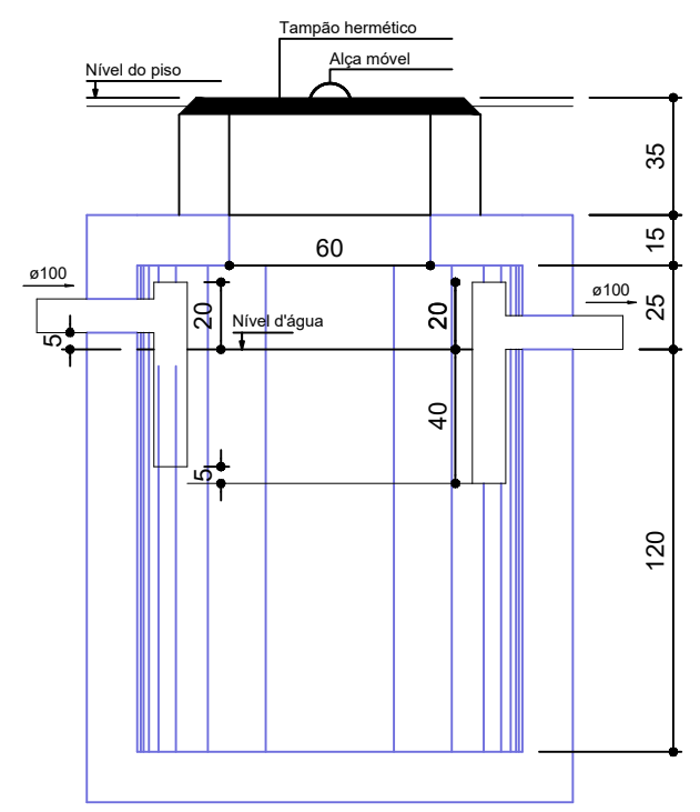
TANQUE SÉPTICO CORTE - escala 1/25
