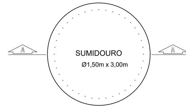
PLANTA BAIXA SUMIDOURO ESCALA - 1/25
