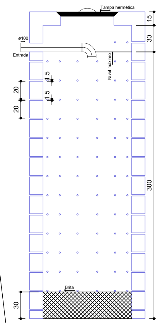
SUMIDOURO CORTE - escala 1/25
