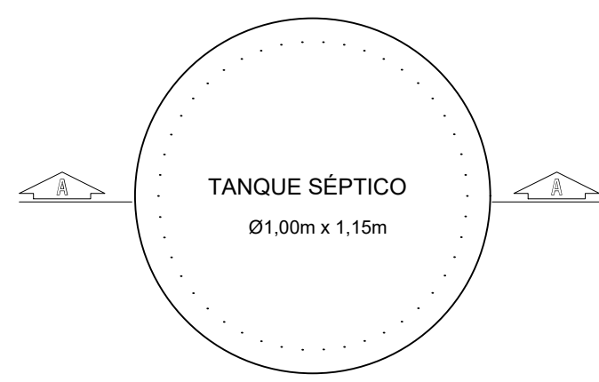
TANQUE SÉPTICO Ø1,00m x 1,15m PLANTA BAIXA TANQUE SÉPTICO ESCALA - 1/25
