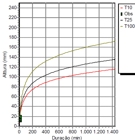
Figura 2 – Curvas Altura/Duração/Frequência
