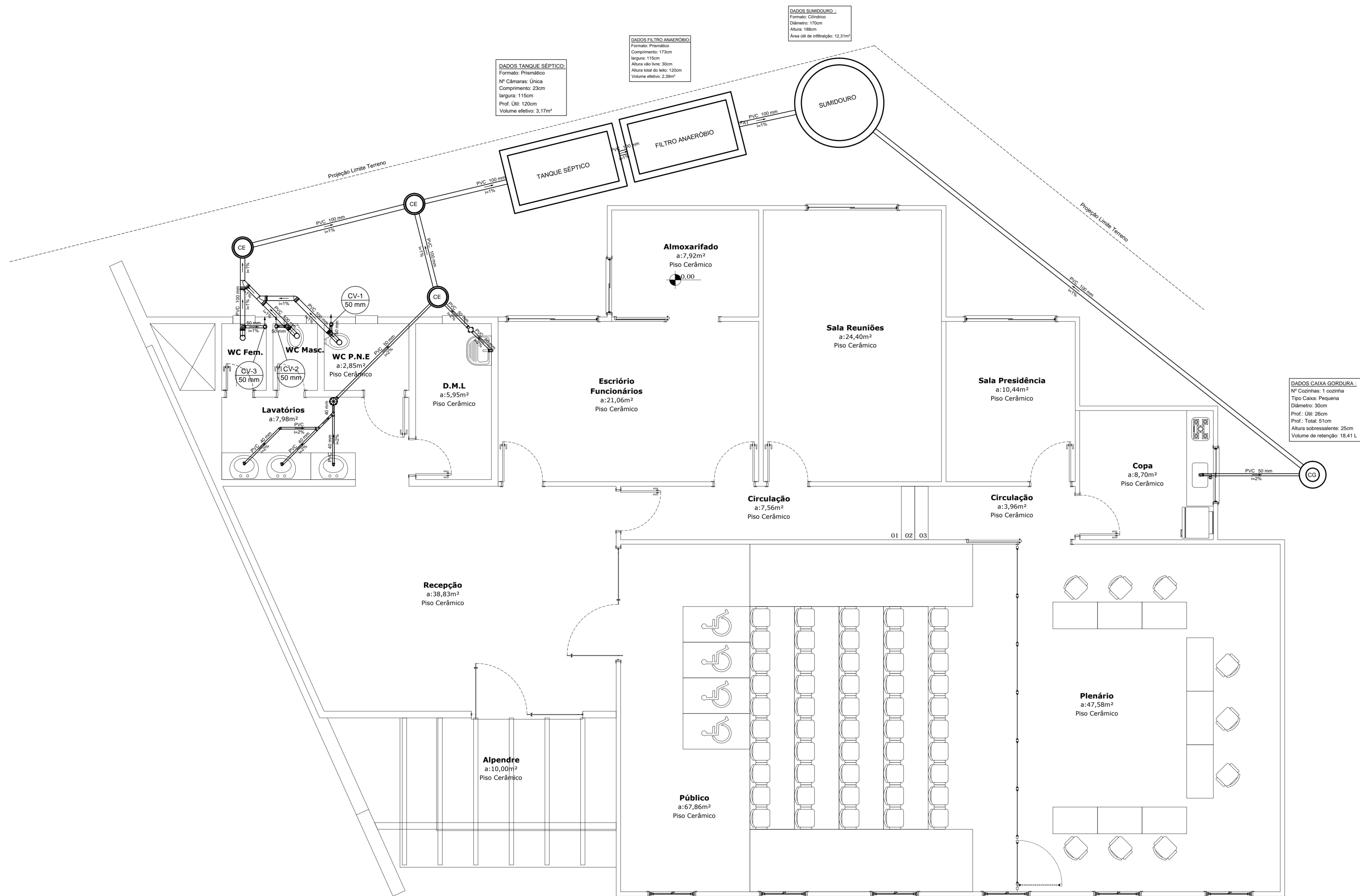
Planta Baixa Área: 288,37 m²
