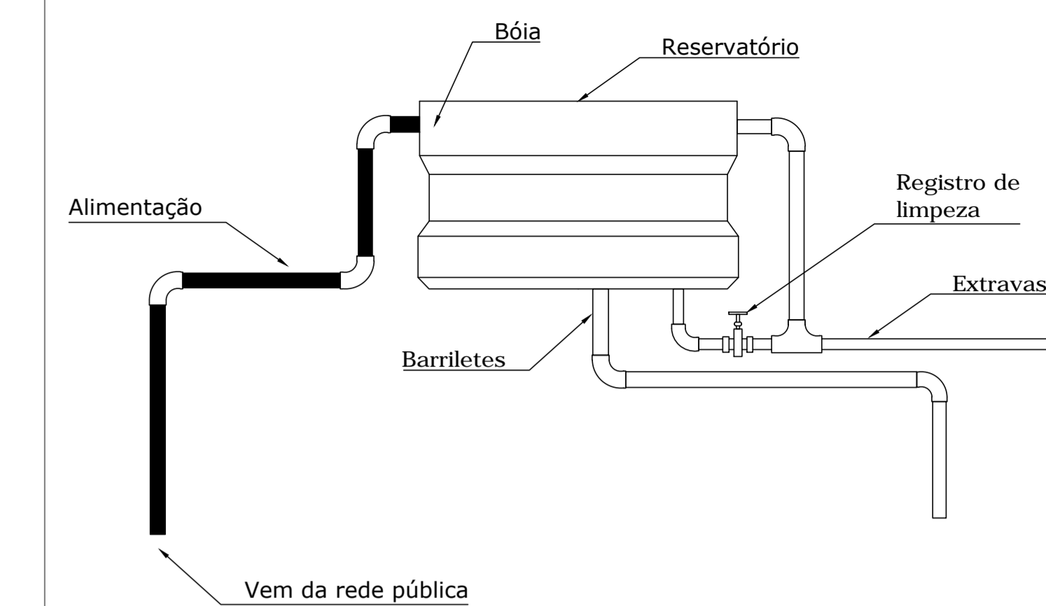
Esquema de tubulação e Limpeza do reservatório S/E
