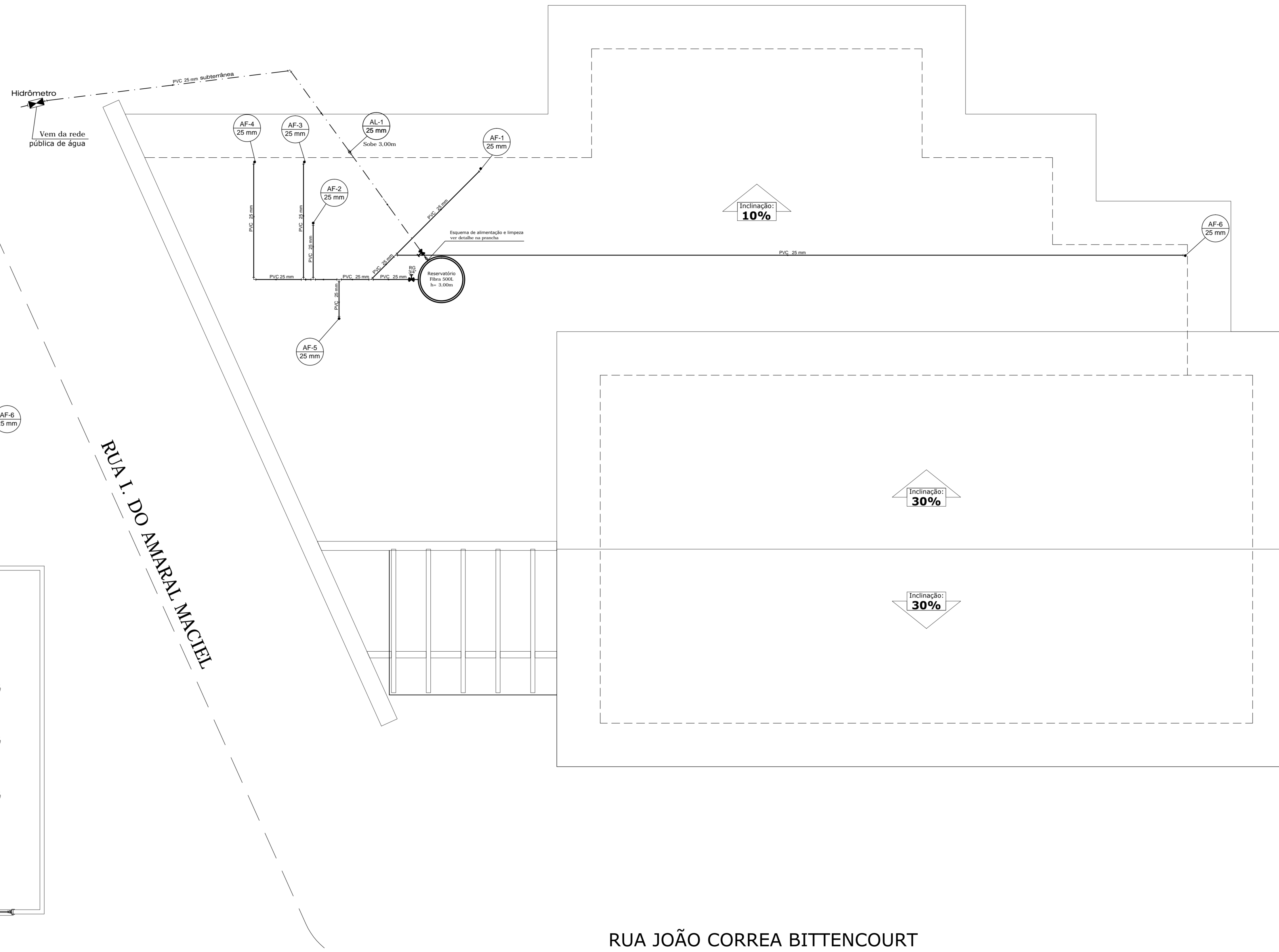
Planta Cobertura- Barrilete e Alimentação Escala 1/50
