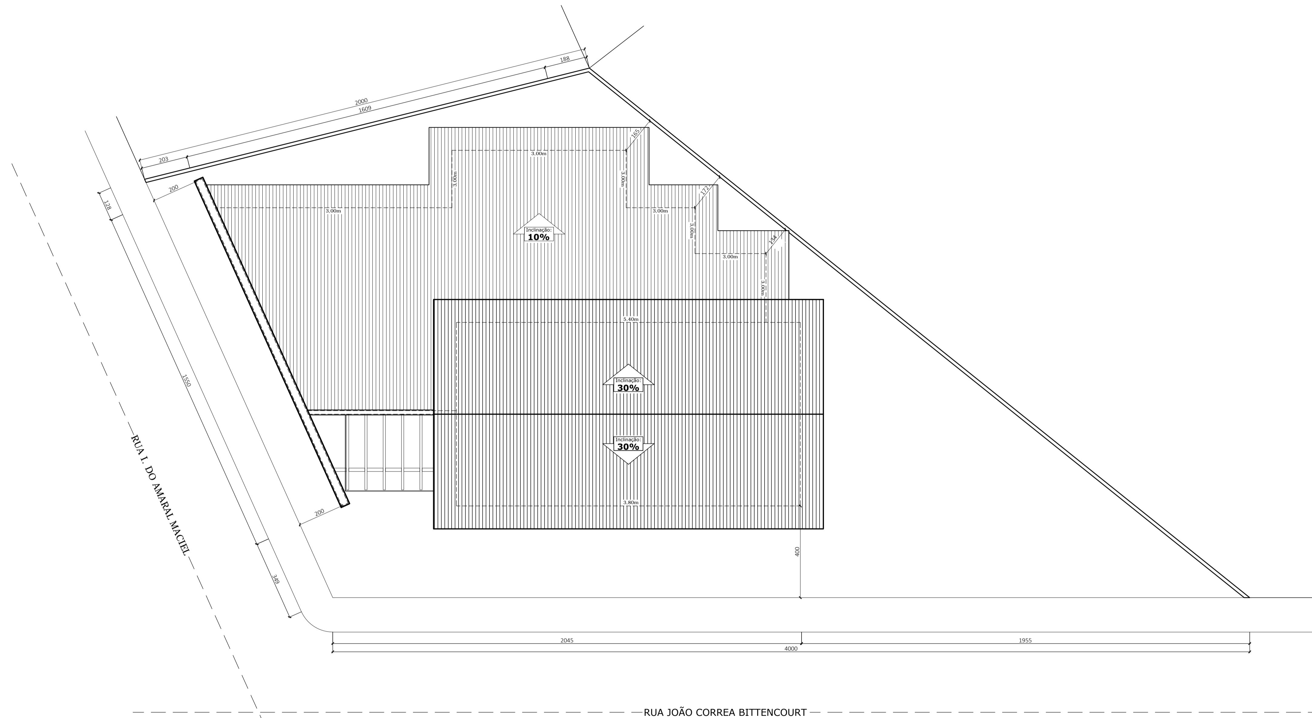
Planta Locação e Cobertura Escala 1/100
