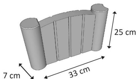
Modelo do guia modular usado no paisagismo.
