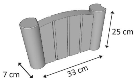
Modelo do guia modular usado no paisagismo.
