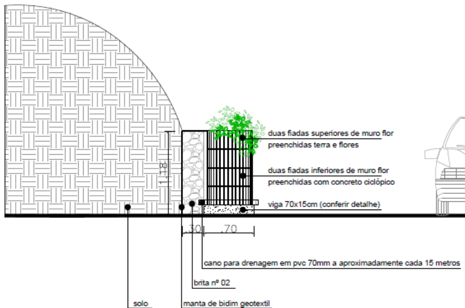
Modelo dos blocos que formam o Muro.
