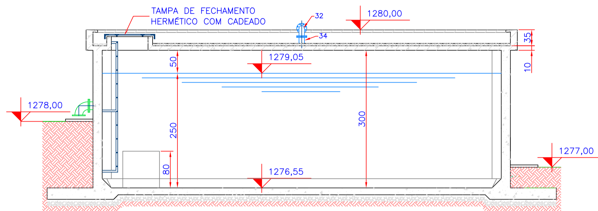
4 CORTE "C-C" ESCALA 1:50
