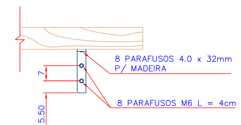
25 DET. DE FIXAÇÃO DA CANTONEIRA ESCALA 1:10
