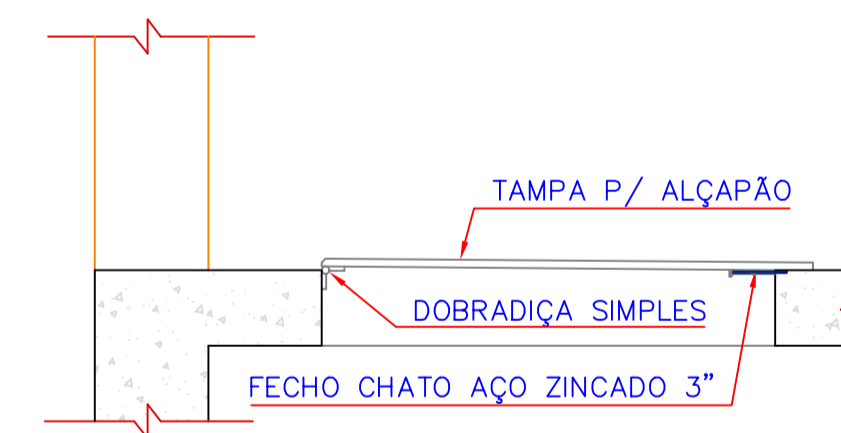
24 DETALHE DO ALÇAPÃO ESCALA 1:10
