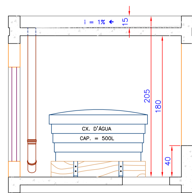
20 CORTE "G - G" ESCALA 1:25
