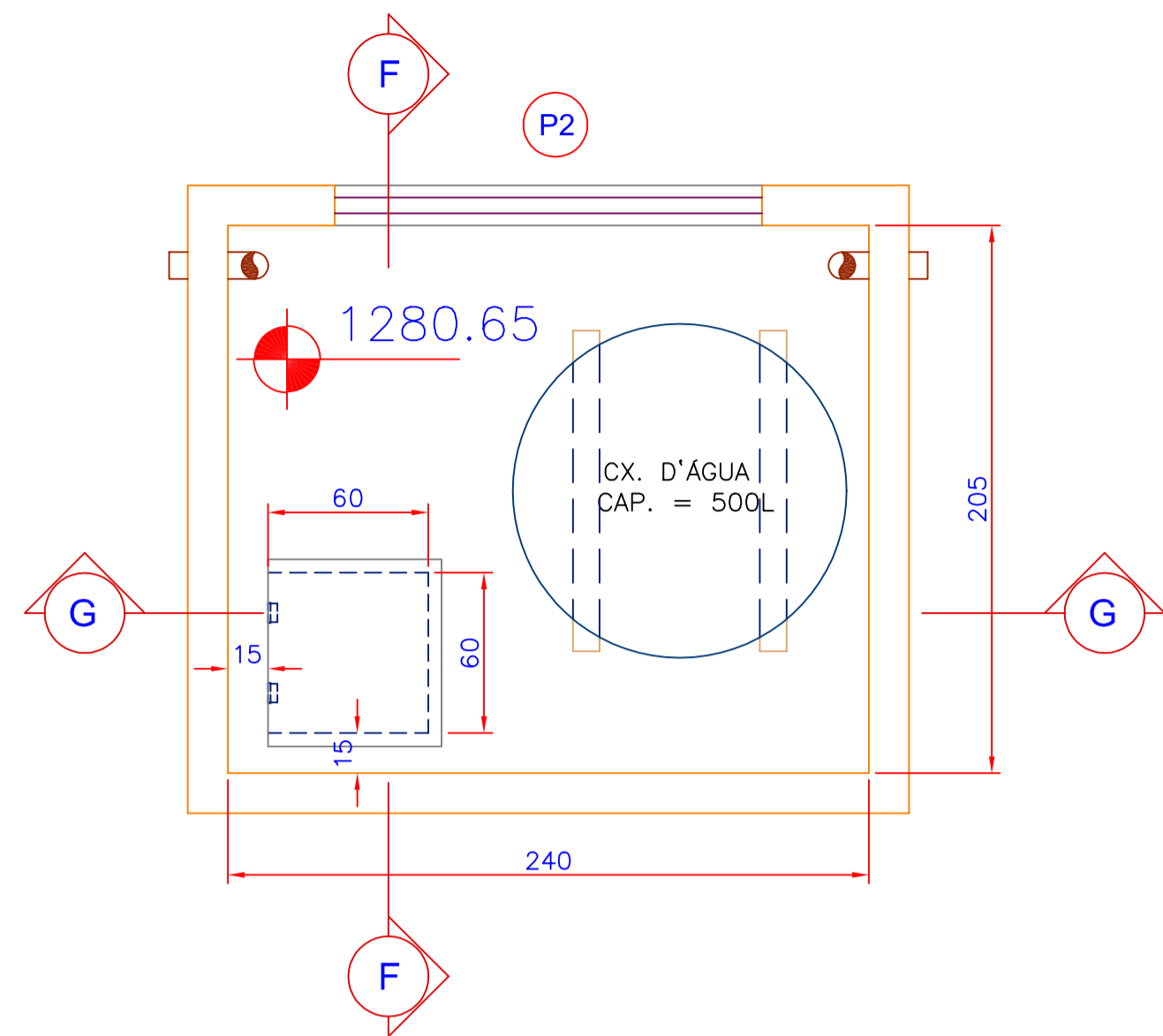
19 PLANTA BAIXA CX. D'ÁGUA ESCALA 1:25
