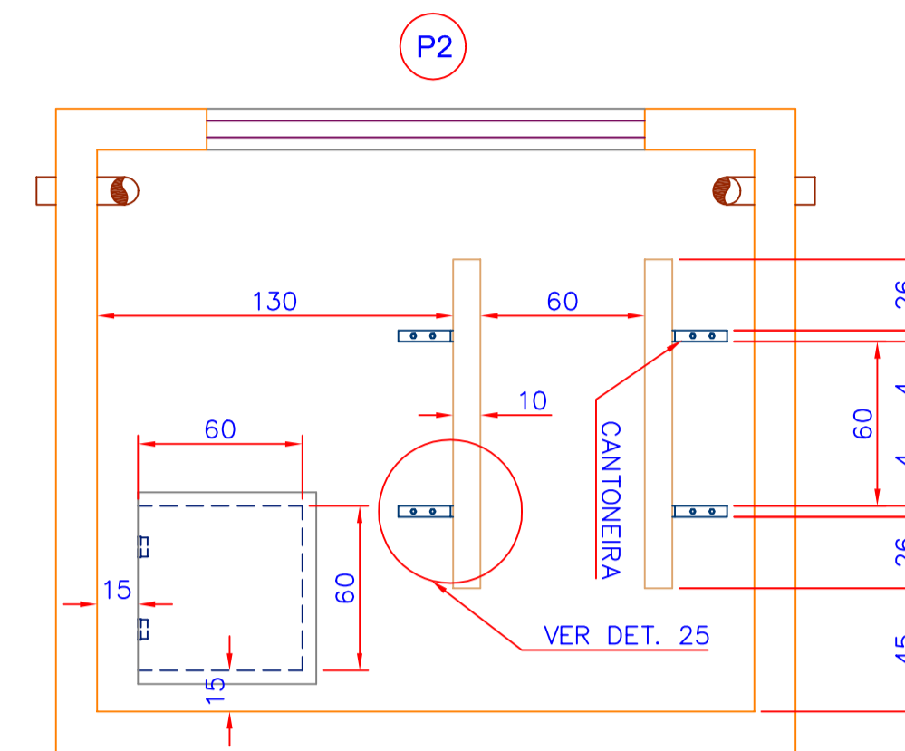
22 CANTONEIRA E SUPORTE CX. D'ÁGUA ESCALA 1:25
