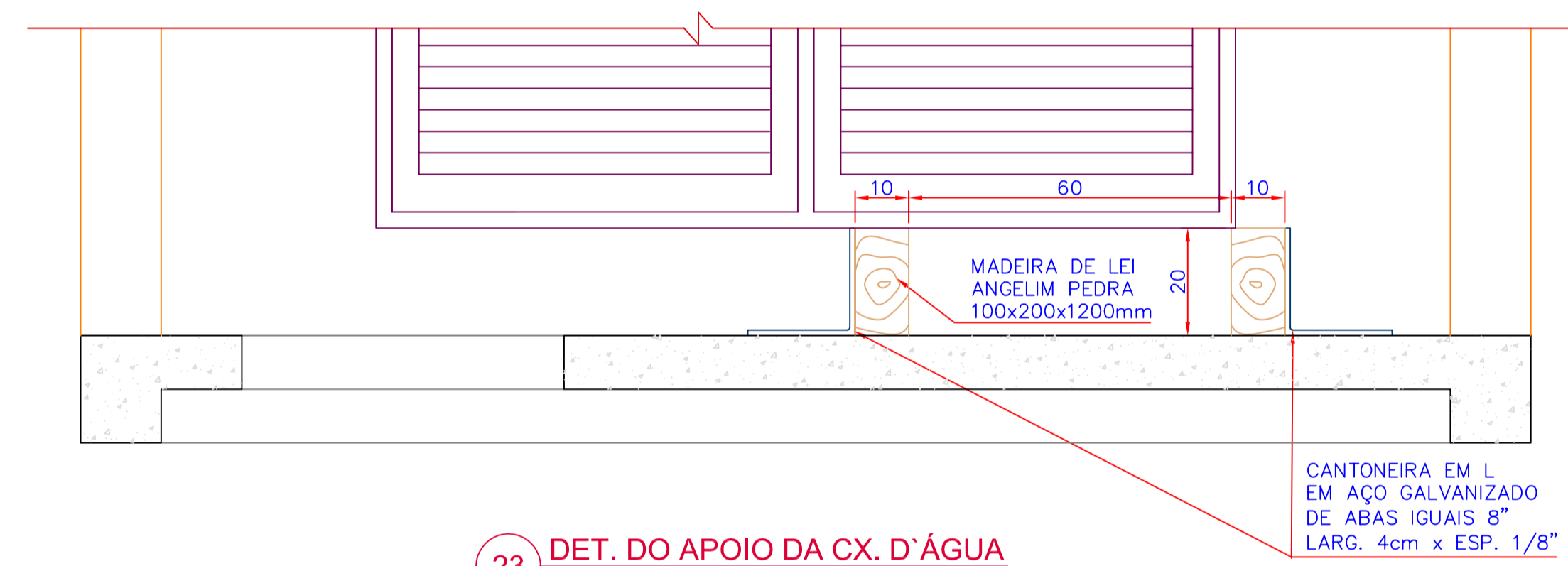
23 DET. DO APOIO DA CX. D'ÁGUA ESCALA 1:10
