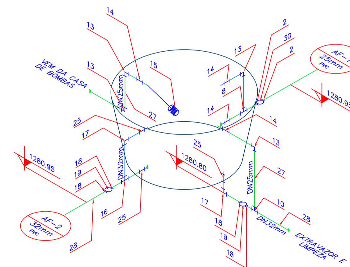
29 ISOMÉTRICO CX. D'ÁGUA ESCALA 1:20
