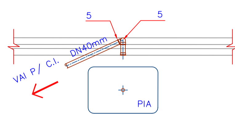
28 ESGOTO PIA ESCALA 1:20
