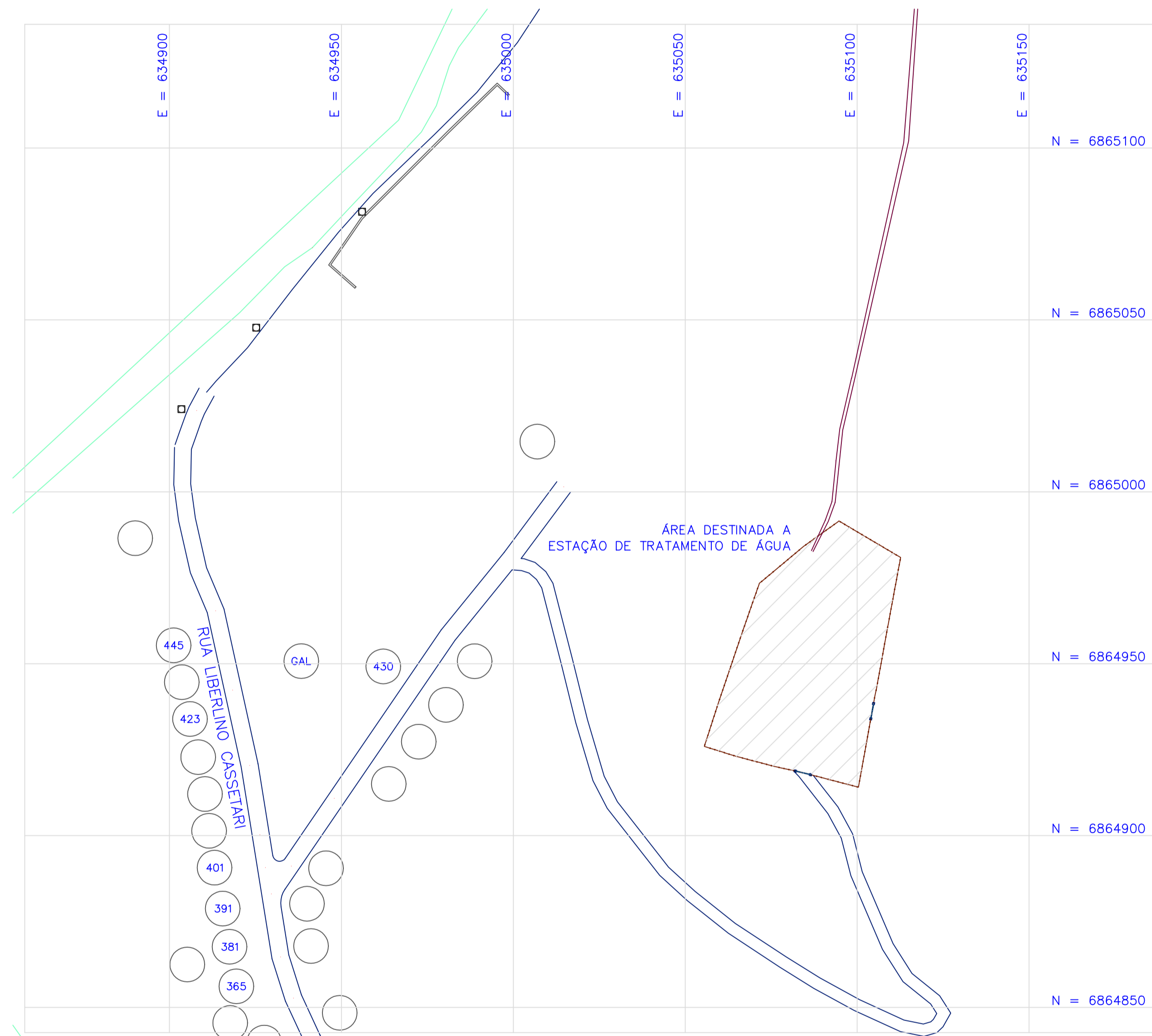
1 SITUAÇÃO ESCALA 1:1000
