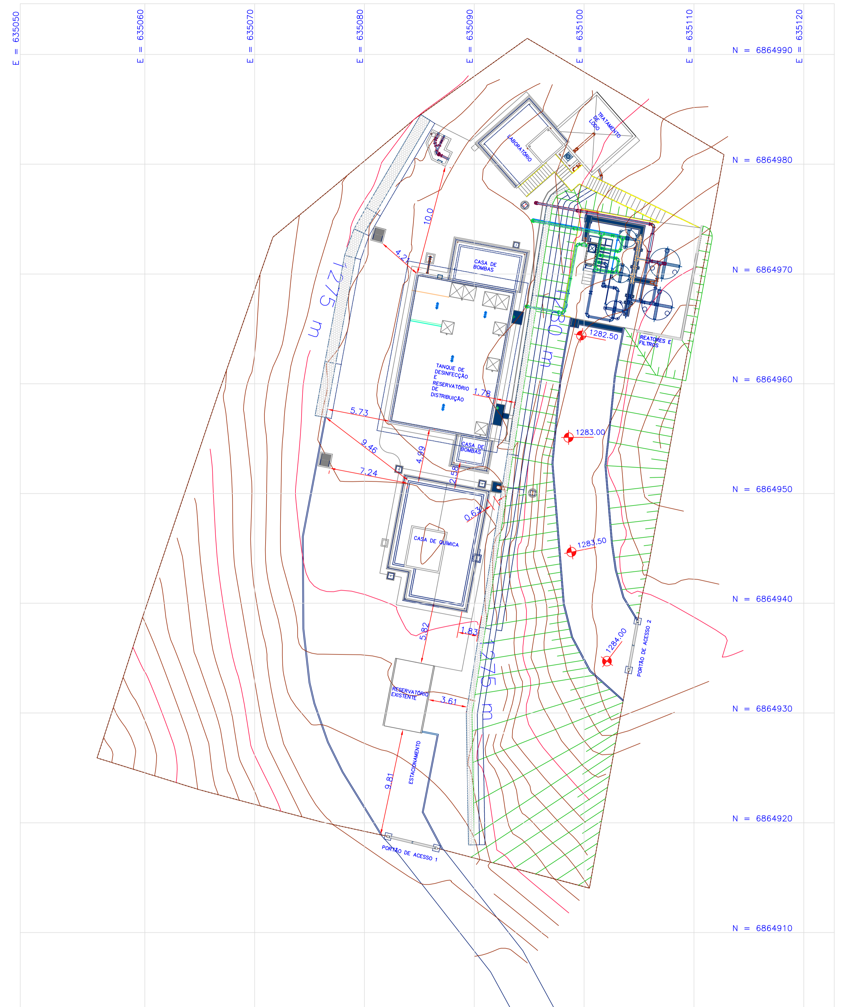
2 LOCAÇÃO ESCALA 1:200
