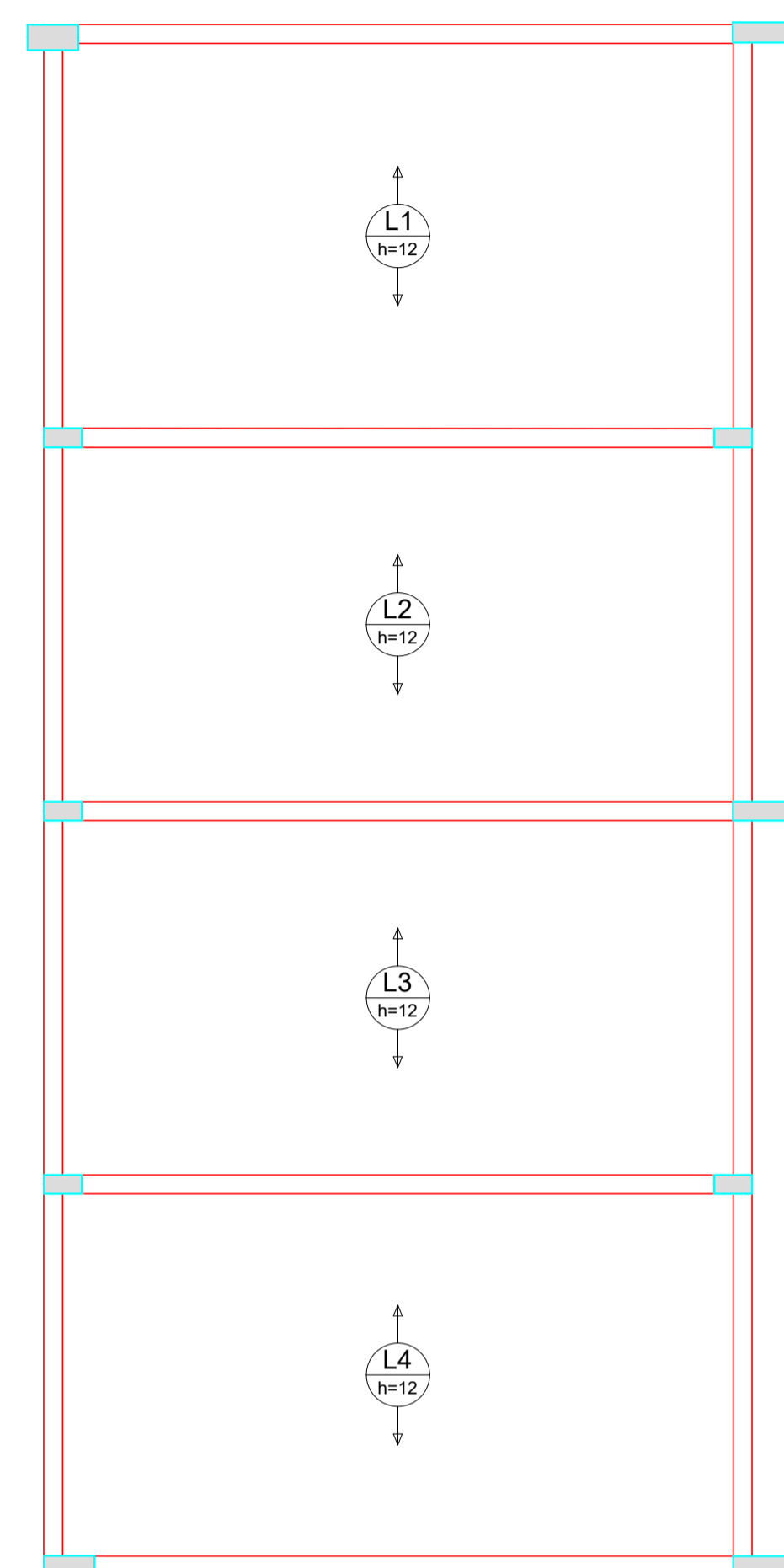
Armação positiva das lajes do pavimento Reservatórios (Eixo Y) escala 1:50
