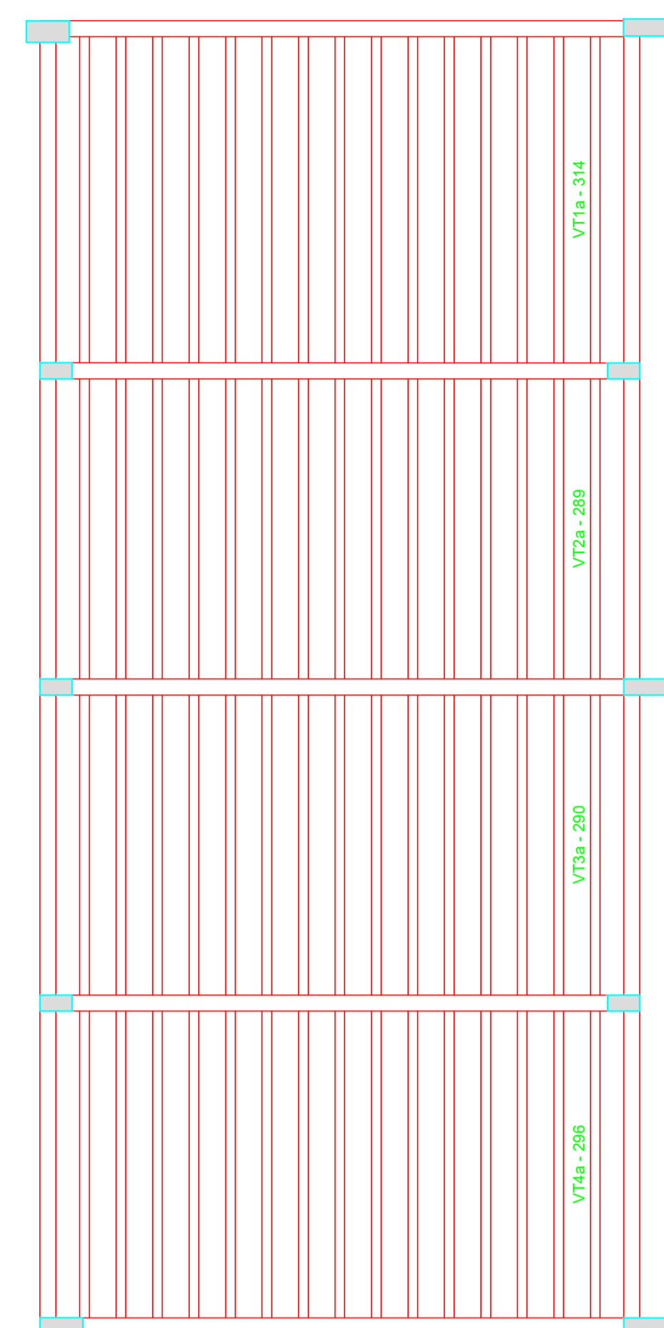
Planta de vigotas pré-moldadas escala 1:50
