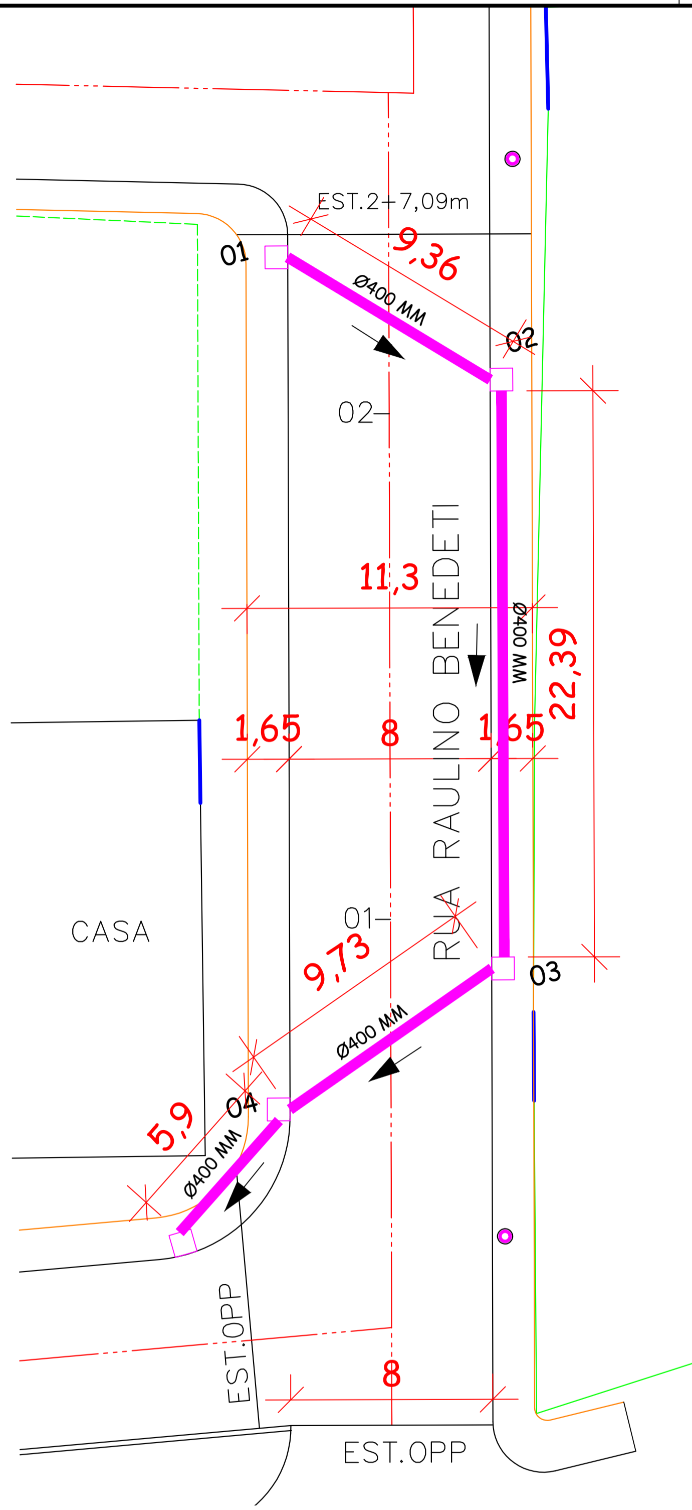
PROJETO DE DRENAGEM PLUVIAL ESCALA 1:150
