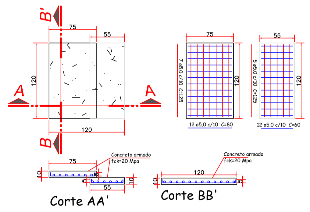
DETALHE - TAMPA BOCA DE LOBO 1,20x1,20 esc 1:30
