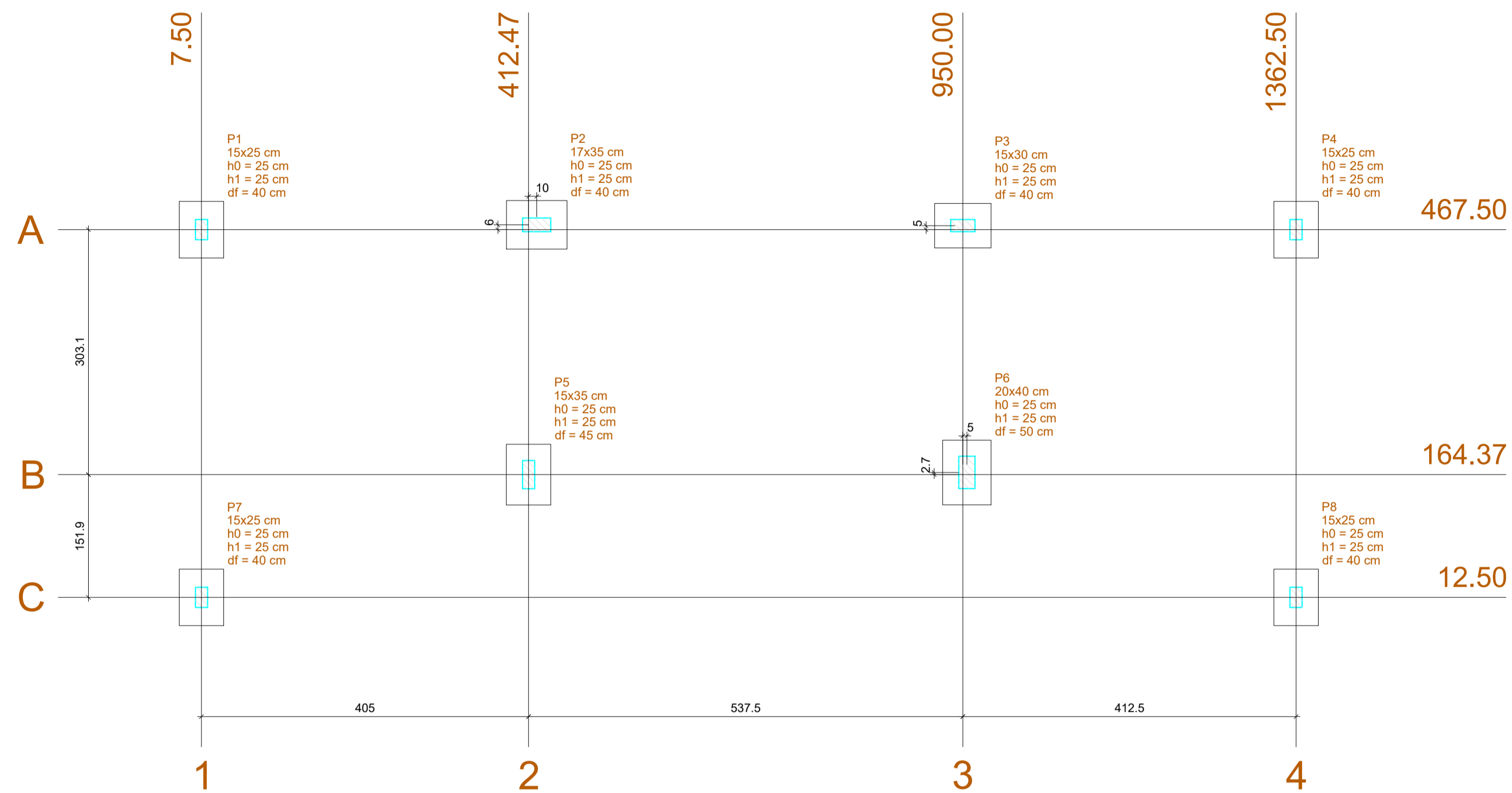
Planta de localização escala 1:50
