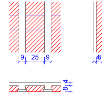
Detalhe 1 (esc. 1:30)
