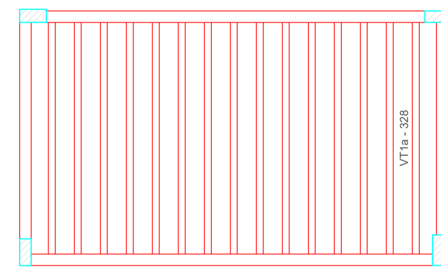
Planta de vigotas pré-moldadas escala 1:50
