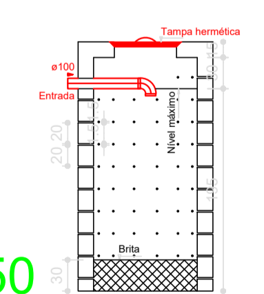
SUMIDOURO CORTE - ESC. 1:50
