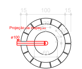
SUMIDOURO PLANTA BAIXA - ESC. 1:50
