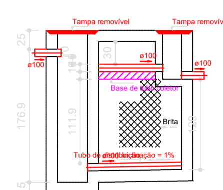
FILTRO ANAERÓBIO CORTE - ESC. 1:50
