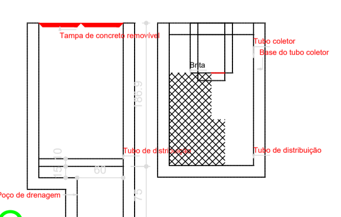
FILTRO ANAERÓBIO CORTES - ESC. 1:50
