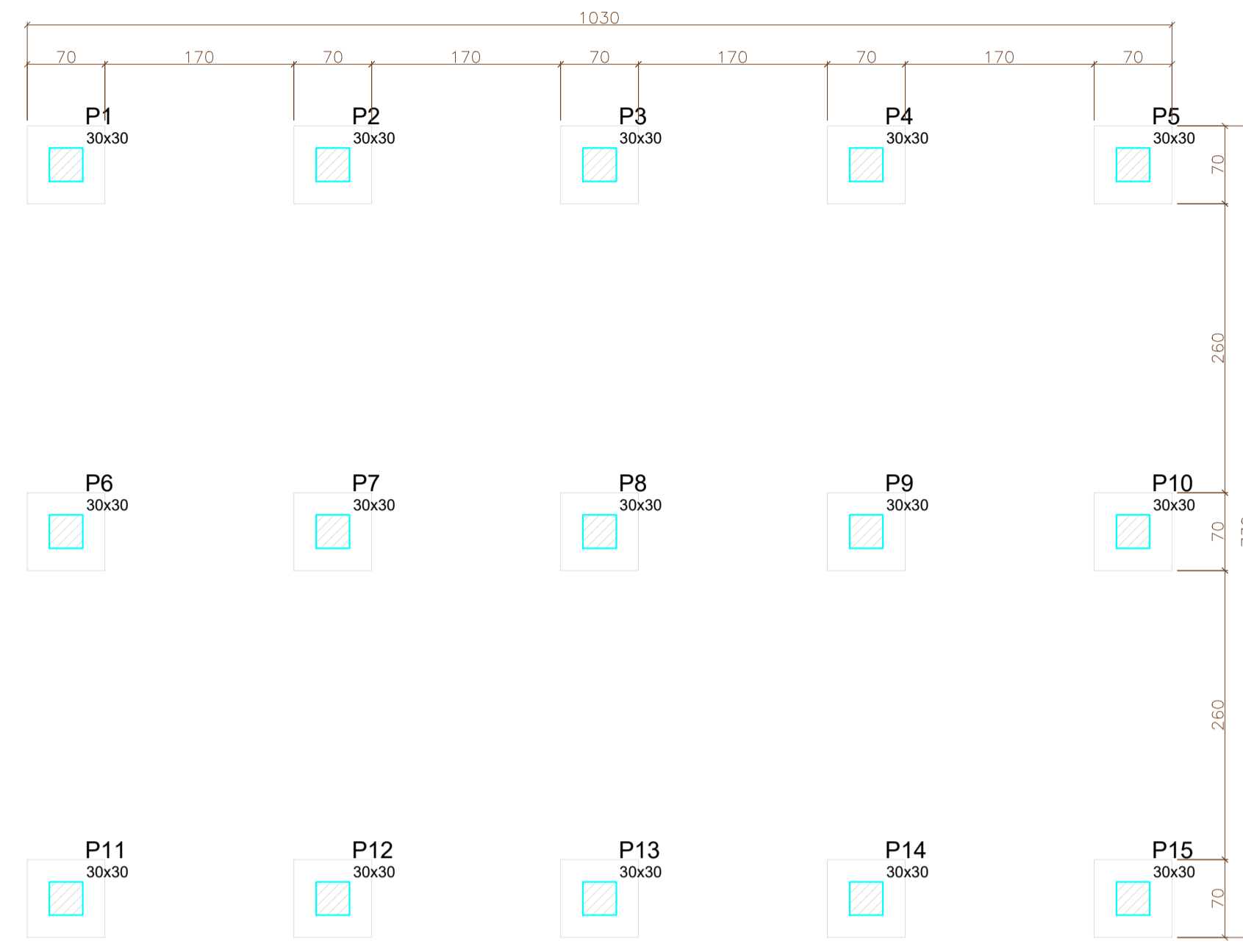
Forma do pavimento fundação escala 1:50
