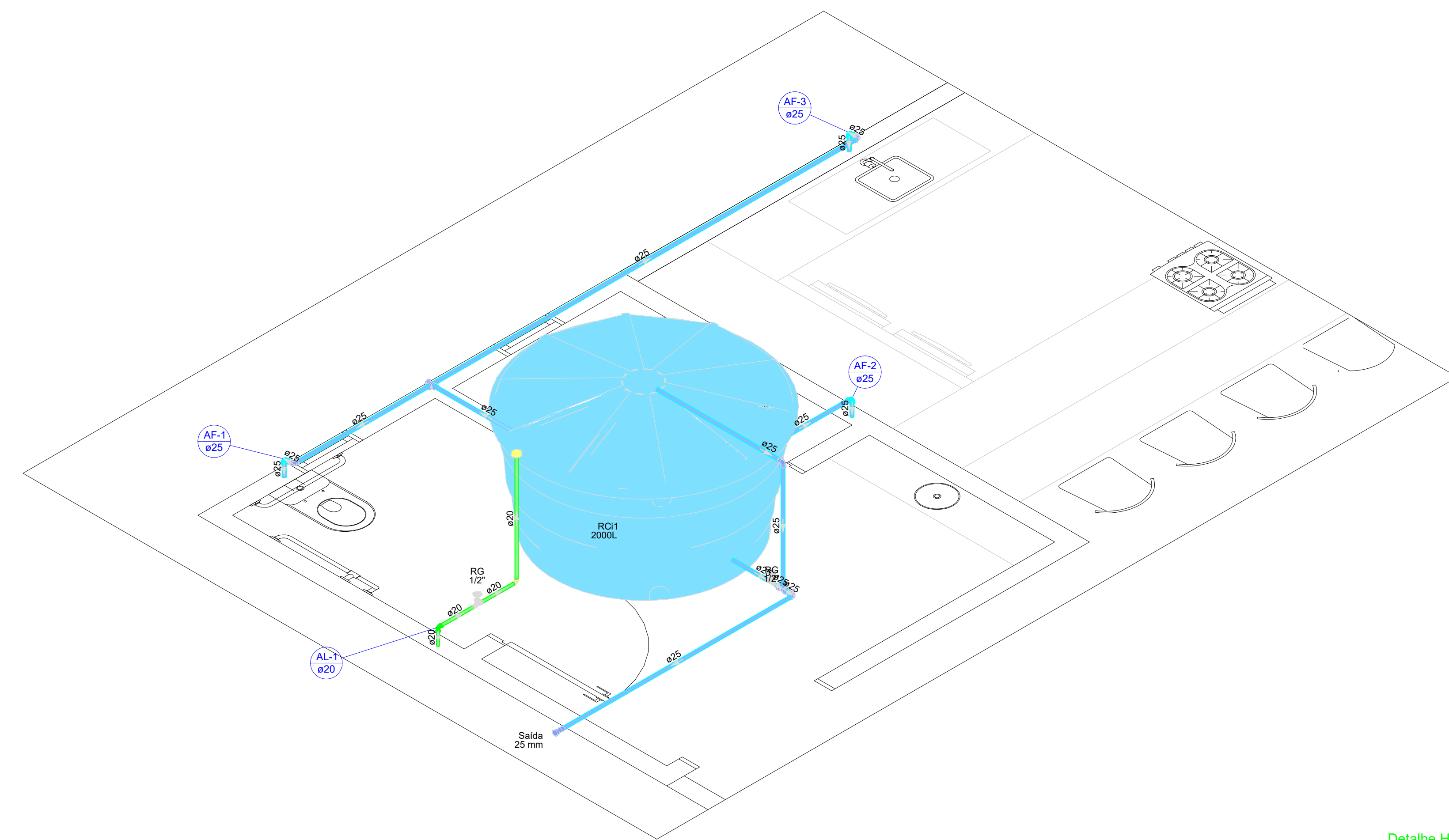
Detalhe H3 Escala 1:50
